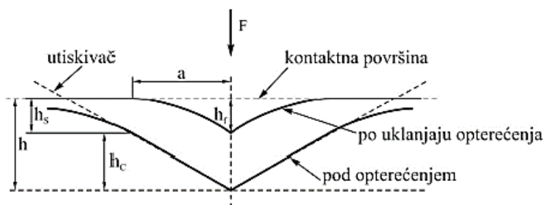
Slika 4 Šematski prikaz ponašanja materijala tokom i po uklanjanju opterećenja
