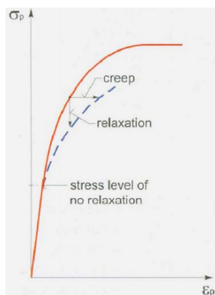
Slika 1 (lijevo): Shematski prikaz puzanja i relaksacije čelika (Ban, 2010. po Navratil, 2006.)
