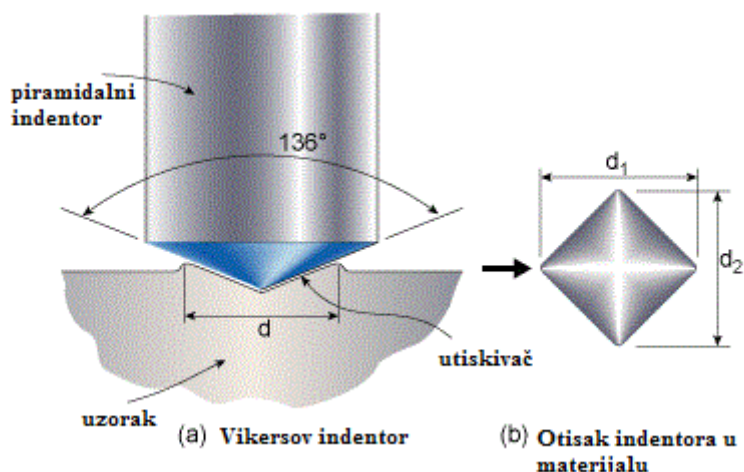
Slika 1 Izgled indentora pri Vickersovoj metodi (a), otisak koji indenter ostavlja na uzorku (b) ( http://www.twi-global.com/ )
