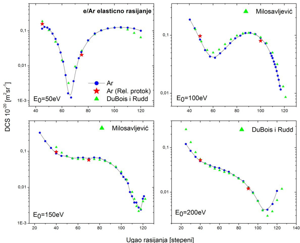
Slika 5. Ugaona zavisnost diferencijalnog presjeka za elastično rasijanje elektrona na atomu argona na različitim upadnim energijama. Finalni eksperimentalni rezultati (krugovi) su predstavljeni zajedno sa vrijednostima dobijenim metodom relativnog protoka (zvjezdice). Trouglovima su predstavljeni rezultati R. D. DuBois-a i M. E. Rudd-a za energije 50eV i 200 eV., odnosno Milosavljevića, za energije upadnih elektrona 100eV i 150 eV.
