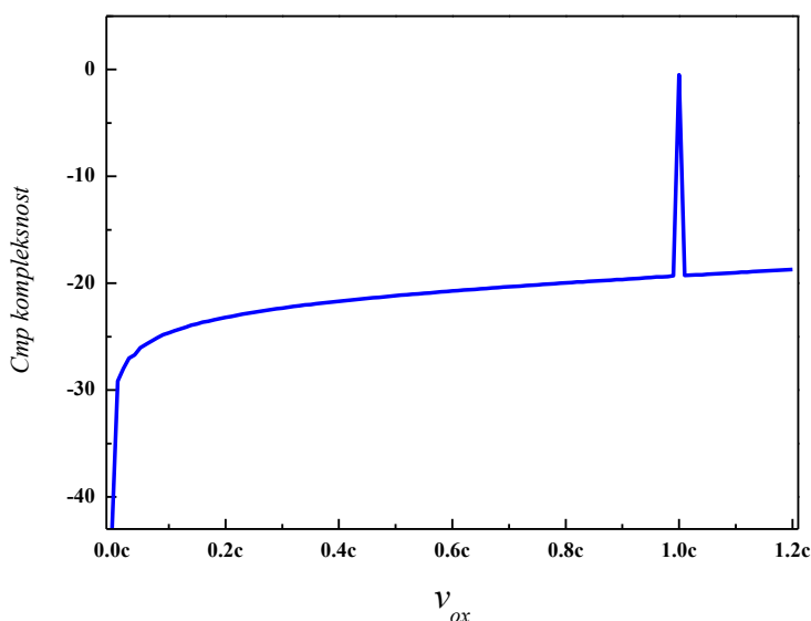
Grafik 3. Cmp kompleksnost pri raznim brzinama v_{0x} za prigušen oscilator
