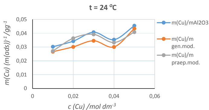
Slika 7. Frojndlihove (Freundlich) adsorpcione izoterme zavisnosti adsorpcije od temperature na 24 °C
