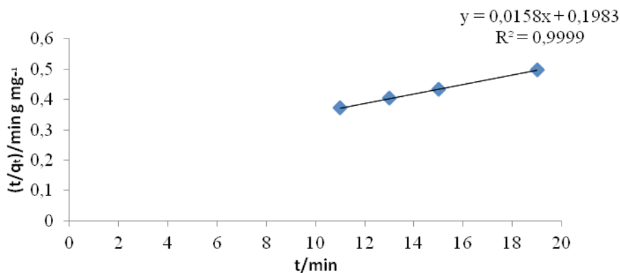
Slika br. 3. Kinetički model pseudo-drugog reda
