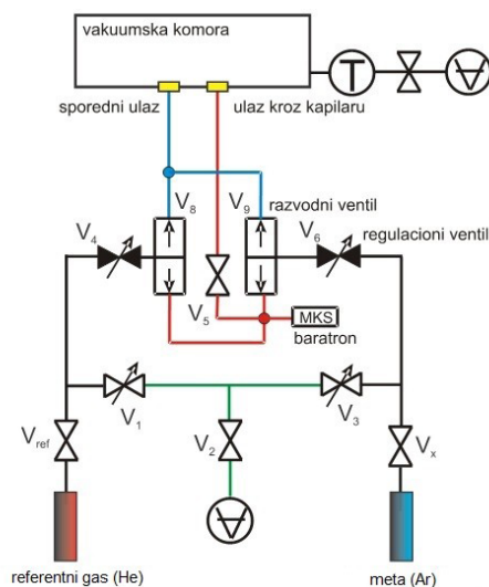
Slika 4. Gasni sistem aparature UGRA
