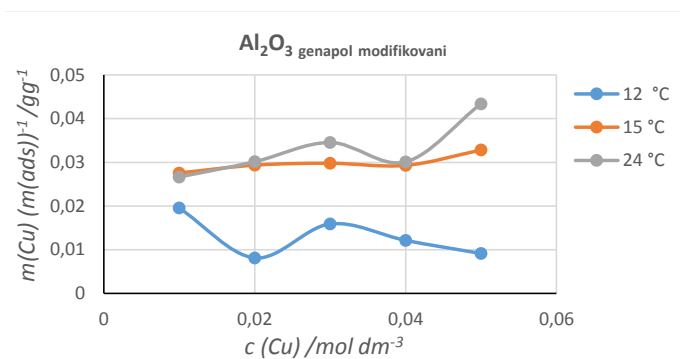
Slika 5. Frojndlihove (Freundlich) adsorpcione izoterme zavisnosti adsorpcije od koncentracije za Al 2 O 3 genapol modifikovani
