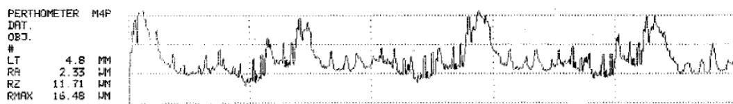
Slika 8. Snimak profila obrađene površine za eksperimentalnu tačku 1.
