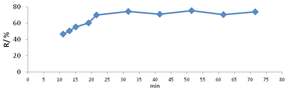
Slika br. 8. Zavisnost % uklanjanja metilen plavog u toku vremena
