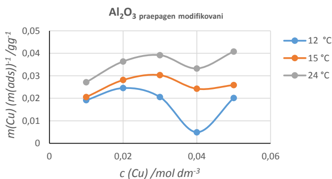
Slika 6. Frojndlihove (Freundlich) adsorpcione izoterme zavisnosti adsorpcije od koncentracije za Al 2 O 3 praepagen modifikovani
