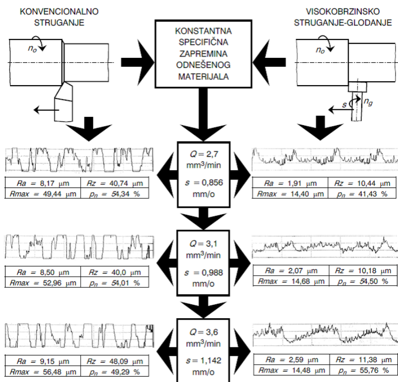
Slika 9. Uporedni prikaz rezultata konvencionalnog struganja i visokobrzinskog struganja-glodanja
