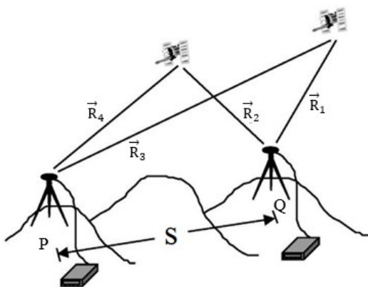
Slika 2. Princip relativnog pozicioniranja primjenom GNSS tehnologije
