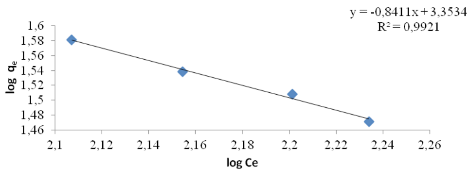
Slika br. 6. Freundlich-ov model izoterme metilen plavog na aktivnom uglju
