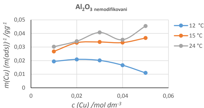
Slika 4. Frojndlihove (Freundlich) adsorpcione izoterme zavisnosti adsorpcije od koncentracije za \text{Al}_2\text{O}_3 nemodifikovani
