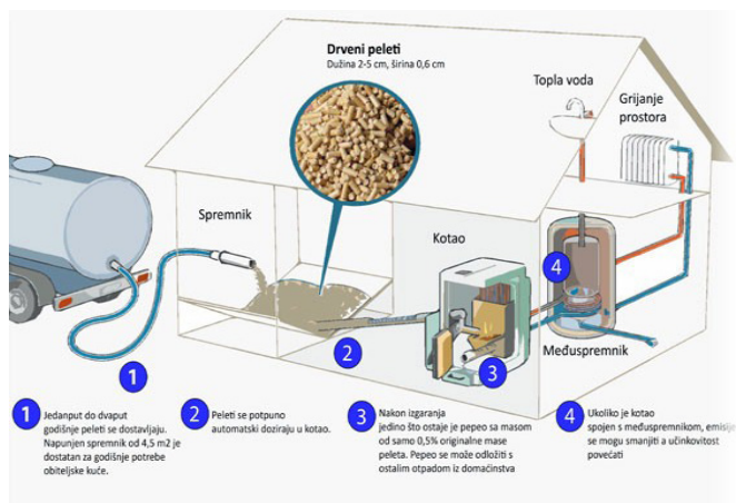
Slika 3. Mogućnost ugradnje na system centralnog grijanja
