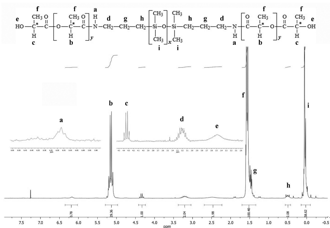
Slika 1. ^1\text{H} NMR spektar uzorka sintetisanog na temperaturi 130^\circ\text{C} i pri koncentraciji katalizatora 1000 ppm
