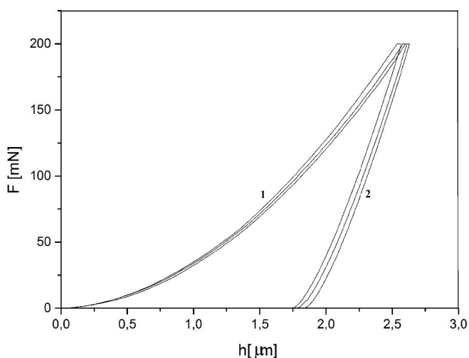
Slika 5 Zavisnost sile opterećenja od dubine otiska (histereza) za stakla iz sistema Fe-Sb-S-I, 1- opterećenje, 2-rasterećenje
